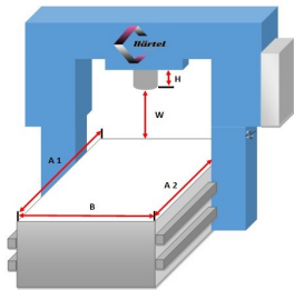
Tisch Portalpresse
