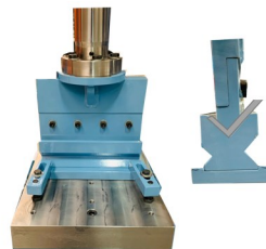
Abkant- Biegewerkzeug
