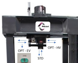
Zylinder seitlich verschiebbar / Verfahrbar je nach Ausführung
